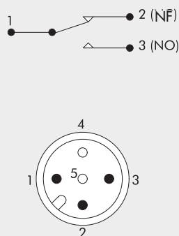
Version avec pressostat
