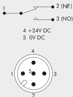
Version avec électropilote et pressostat
